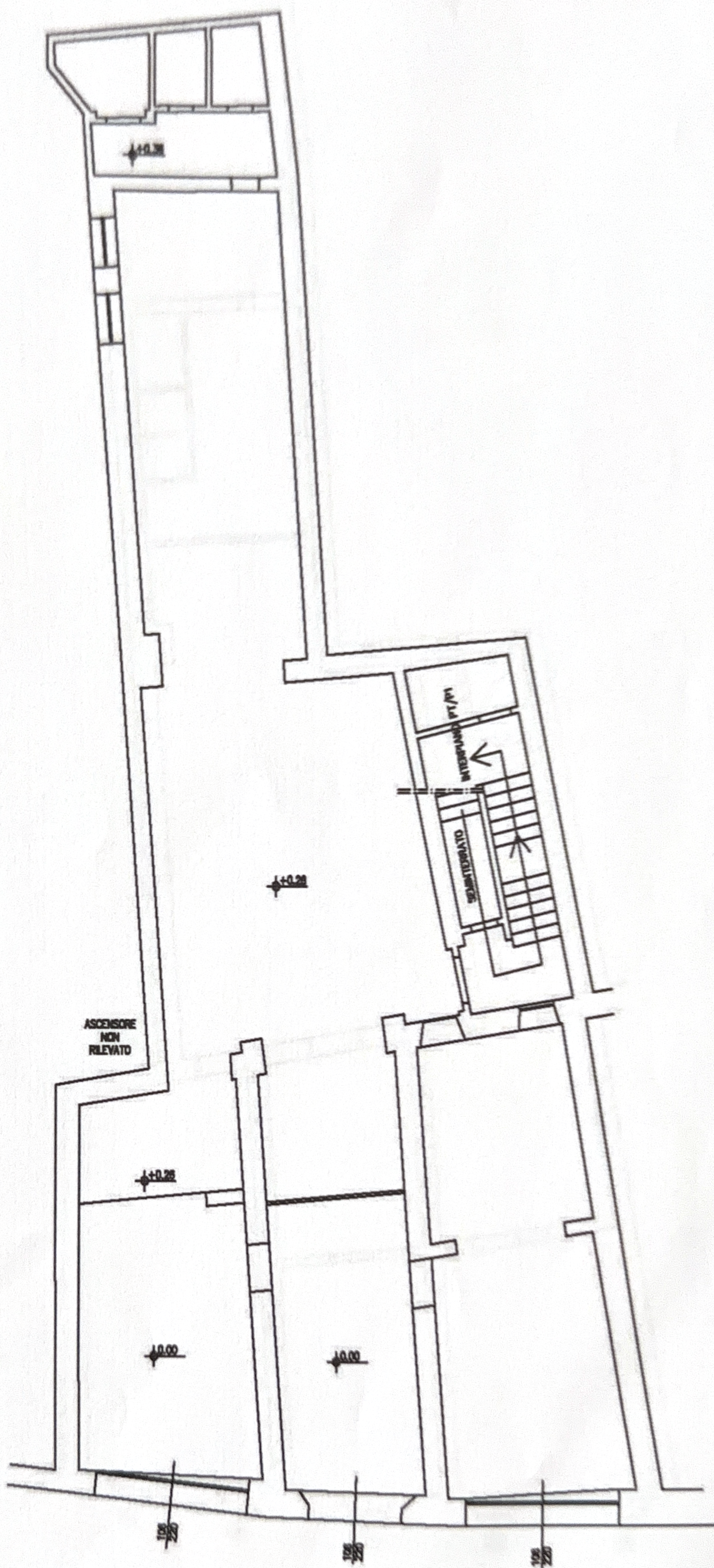
PIANO TERRA - INTERPIANO PT/P1 SUPERFICIE 32,00 M2
